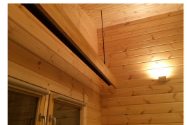
ブレース吊り(ログハウス)
